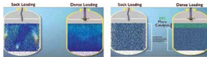
شکل ۲: مقایسه بارگذاری متراکم یکنواخت و بارگذاری جوراب
